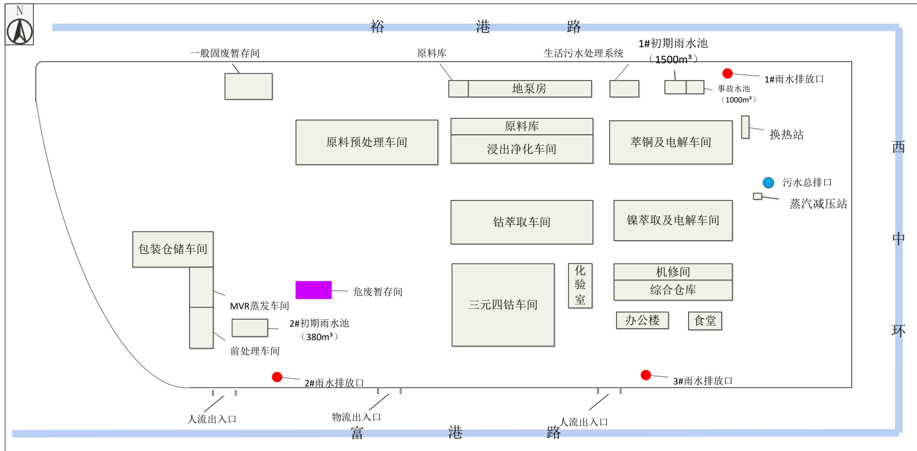
附图 3: 厂房平面布置图
