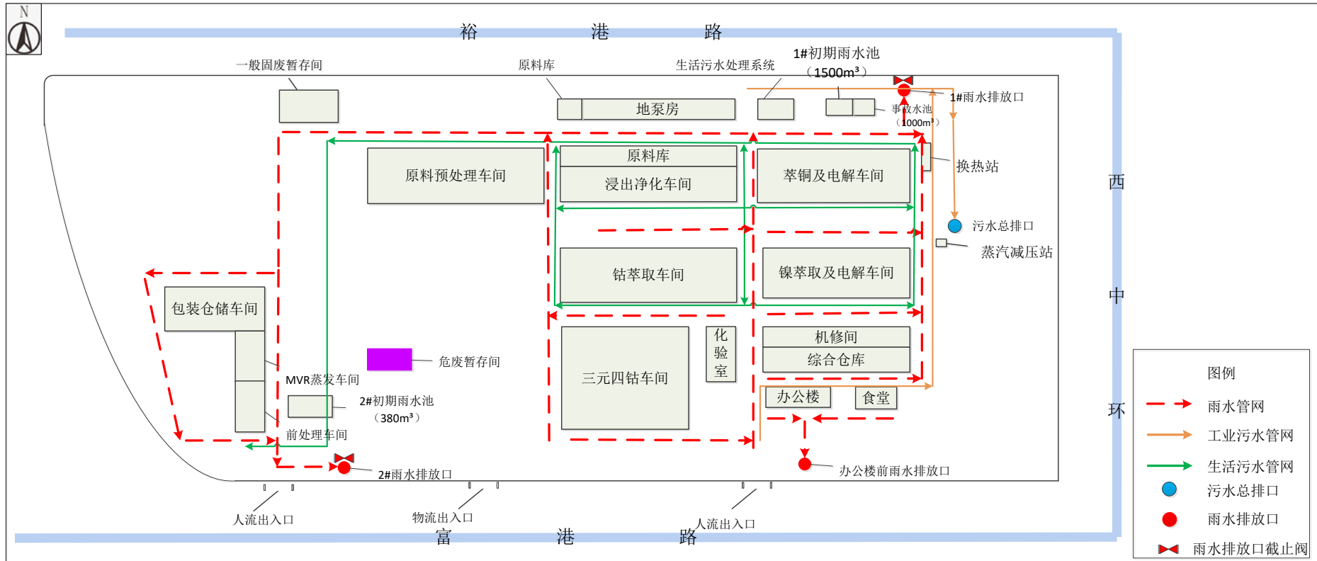
附图 4: 厂区雨污水管网图
